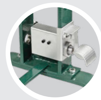
Fußbedienter Schnellhub des Kolbens mit Druckluft! (FP 25/FP 30)
